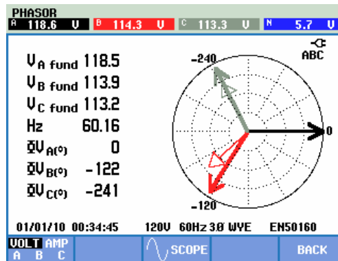
Abbildung 6-3. Vektordiagramm für den korrekt angeschlossenen Analysator
