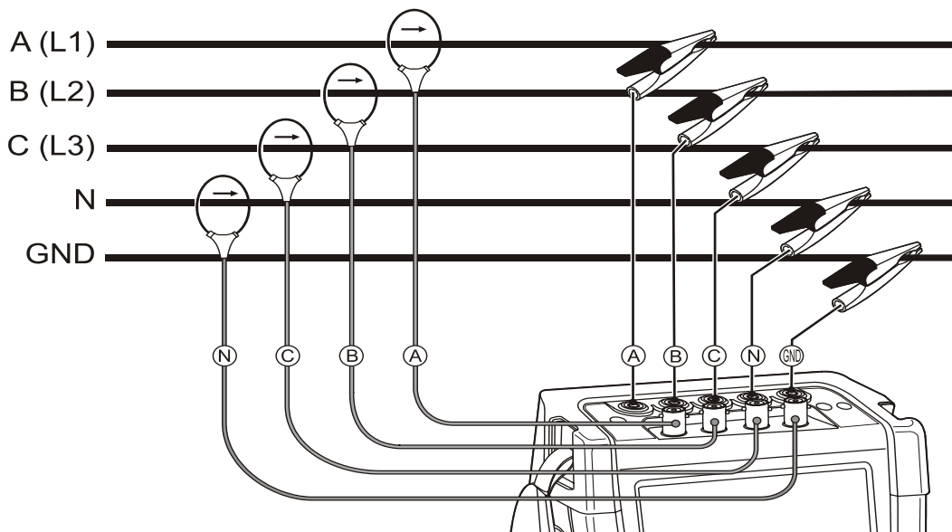
Abbildung 6-2. Anschluss des Analysators an dreiphasige Stromverteilungssysteme
