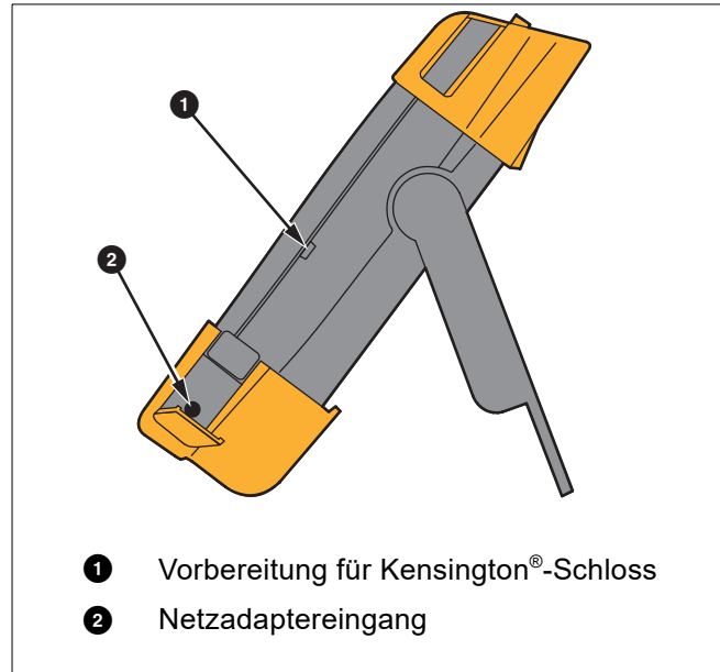
Abbildung 43. Aufstellbügel
