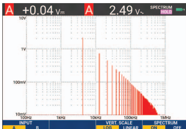
Abbildung 9. Spektralmessung
