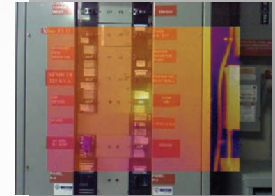
50 % Überblendung, Bild-in-Bild-Modus
