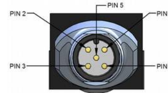
Steckeransicht Sensor
