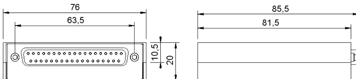
Abbildung 1: Abmessungen GSV-4CAN
