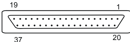
Abbildung 2: 37-pol. Sub-D Buchse
