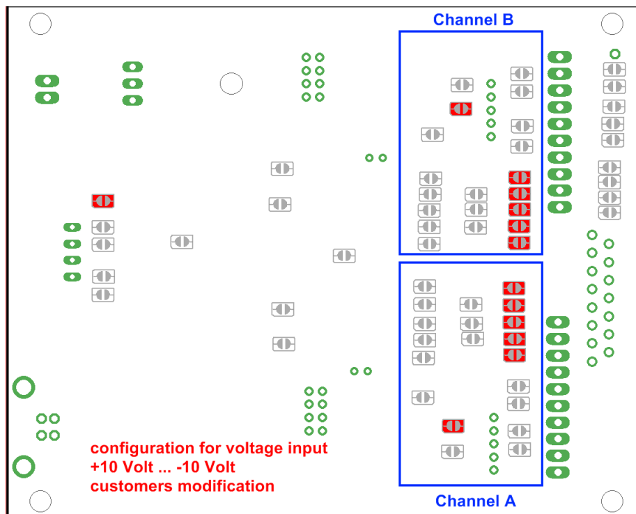
Abbildung 8: Spannungseingang +-10 Volt
