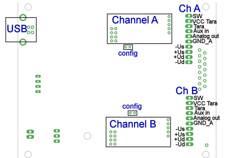
Abbildung 4: Pinbelegung, Platinenoberseite
