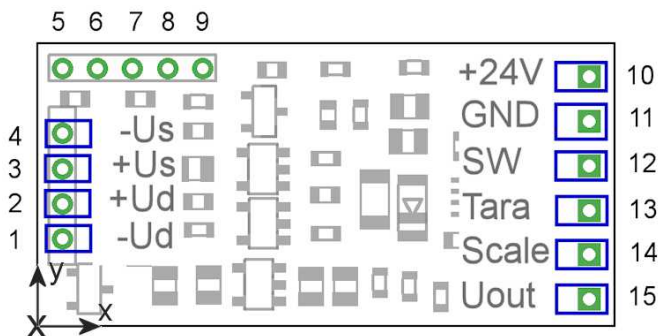
Abbildung 3: Anschlussbelegung, Ansicht: Oberseite
