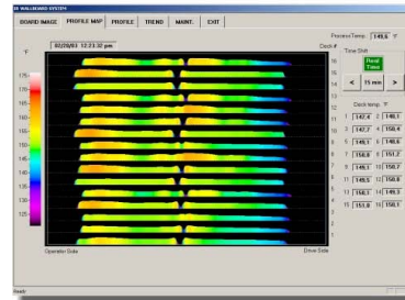
Gemitteltes Temperaturprofil von Gipsplatten (für 16 Trockner dargestellt)
