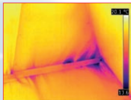
Thermogramm bei Unterdruck während einer BlowerDoor-Messung: Die Leckagen in der Gebäudehülle werden deutlich sichtbar.
