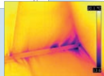
Thermogramm bei Unterdruck während der BlowerDoor-Messung
