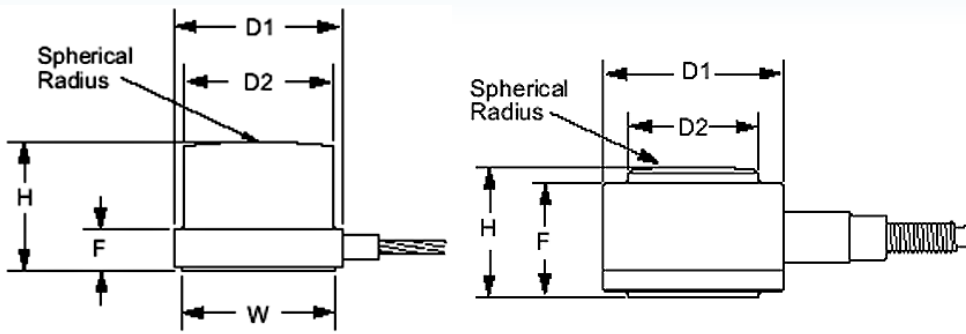
Cable-B shielded Teflon with S ring strain relief / Geschirmtes Kabel mit S Ring Zugentlastung
