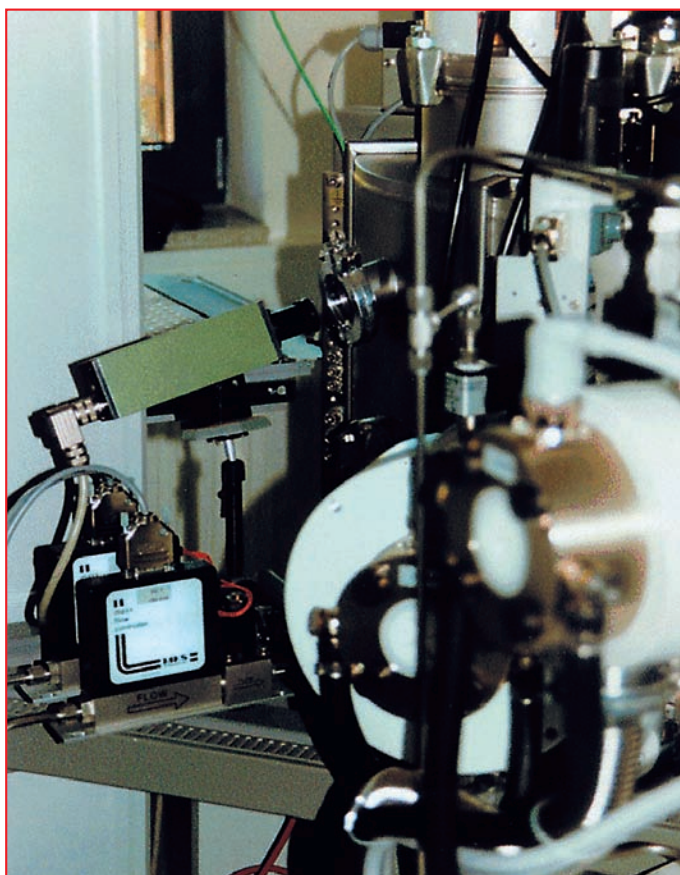
Bild 1 Anwendungen bei Vakuumkammern erfordern häufig angepasste Pyrometerlösungen mit speziellen Optiken, Messwellenlängen und Softwareschnittstellen.
