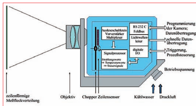
Bild 2 Prinzipieller Aufbau des Kamerakopfes am Beispiel einer Linienkamera.
