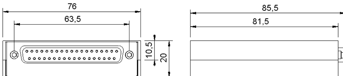
Abbildung 1: Abmessungen GSV-4CAN
